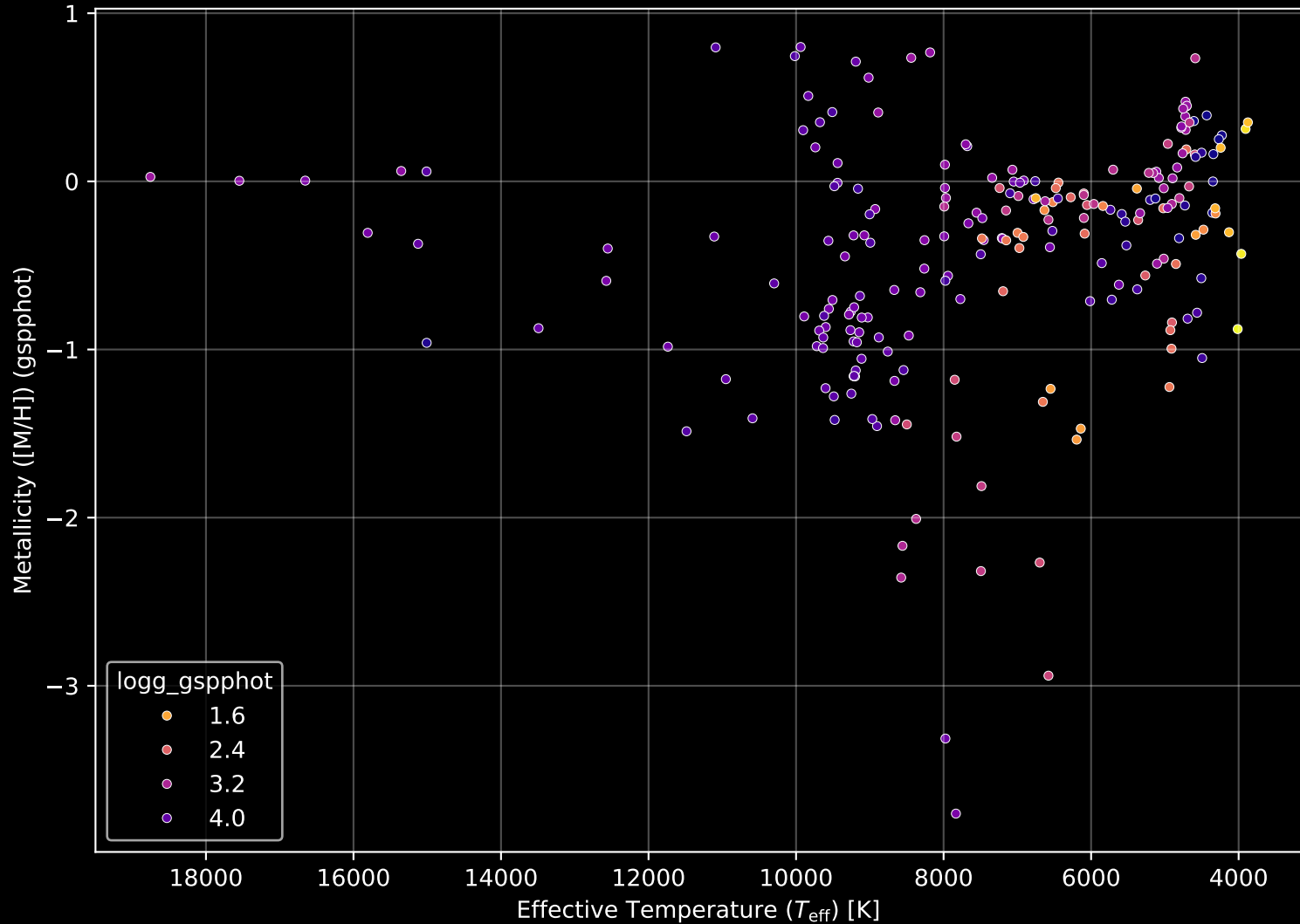
APOGEE DR17 Field: [109+00] Stellar Population Parameters (n= 223)
